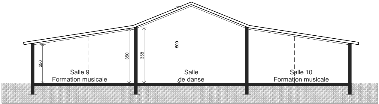
COUPE AA
